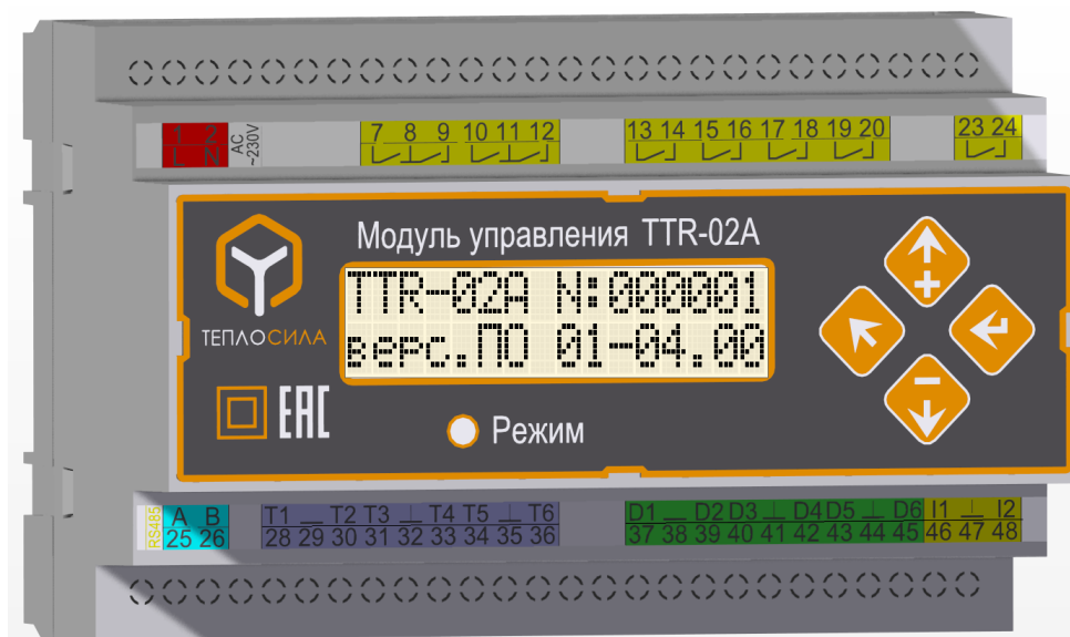
Рисунок 1 – Внешний вид модуля управления TTR-02A
