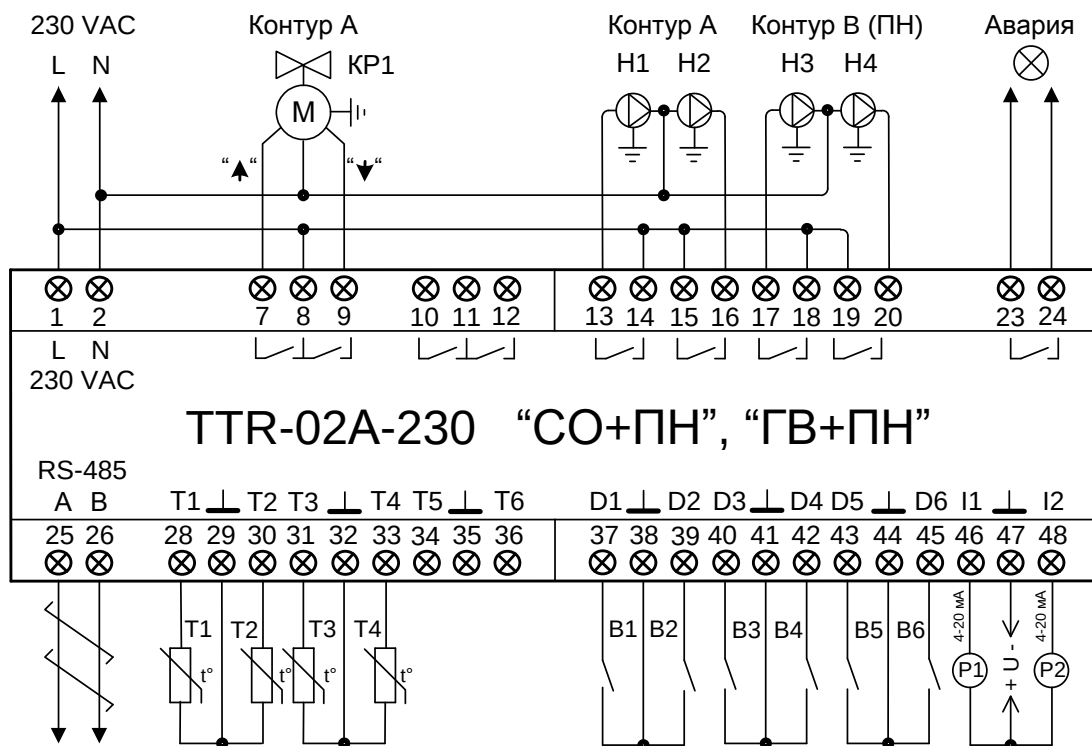
Рисунок В.4 – Схема подключений ТТR-02A-230 для одноконтурной СО или ГВС с дополнительным контуром повысительных насосов (ПН)
