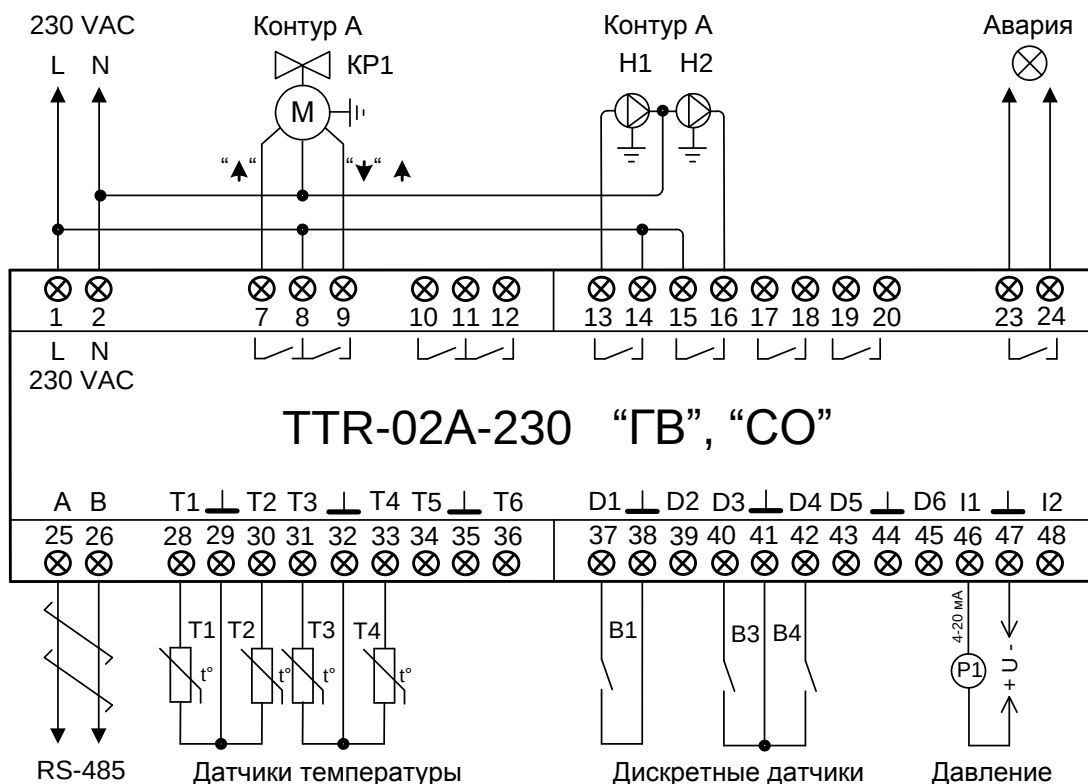
Рисунок В.2 – Схема подключений TTR-02A-230 одноконтурной СО или ГВС для схемы 2 и 3 дискретных входов D1...D6 (см. таблицу В.2)
