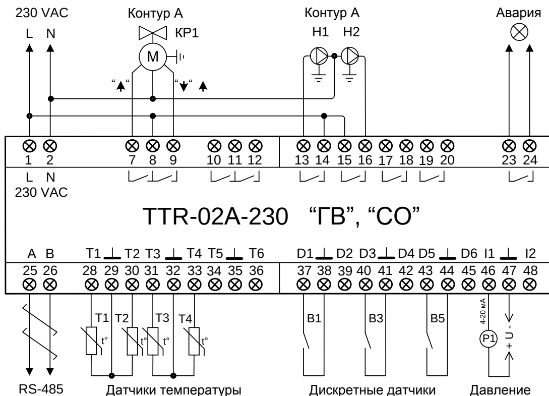
Рисунок В.1 – Схема подключений TTR-02A-230 одноконтурной СО или ГВС для схемы 1 дискретных входов D1...D6 (см. таблицу В.2)
