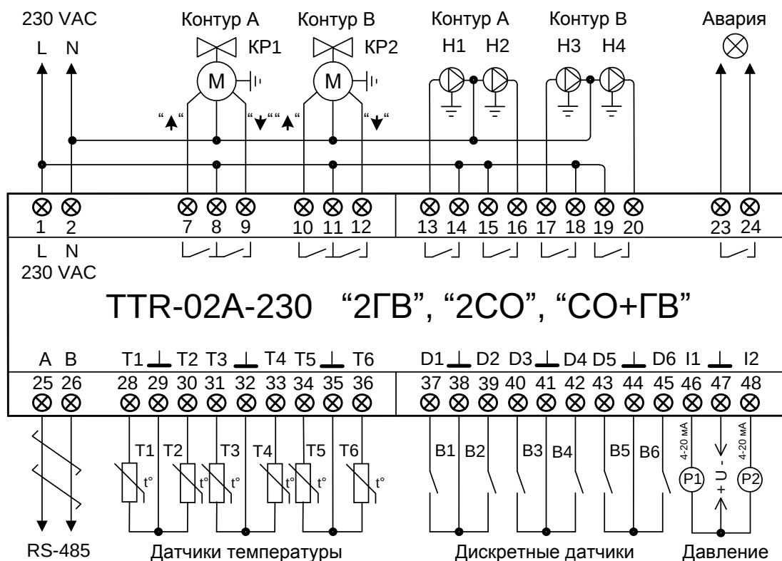
Рисунок В.3 – Схема подключений ТТR-02A-230 для двухконтурной СО и ГВС
