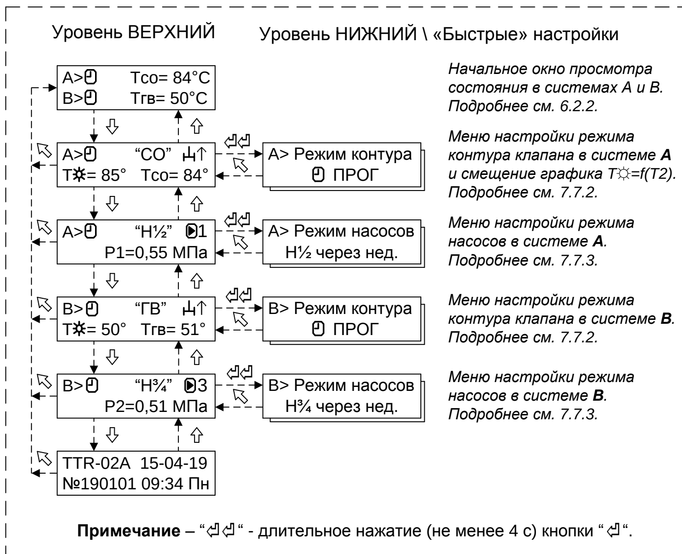
Рисунок 22 – Структура меню «быстрой» настройки режима работы
