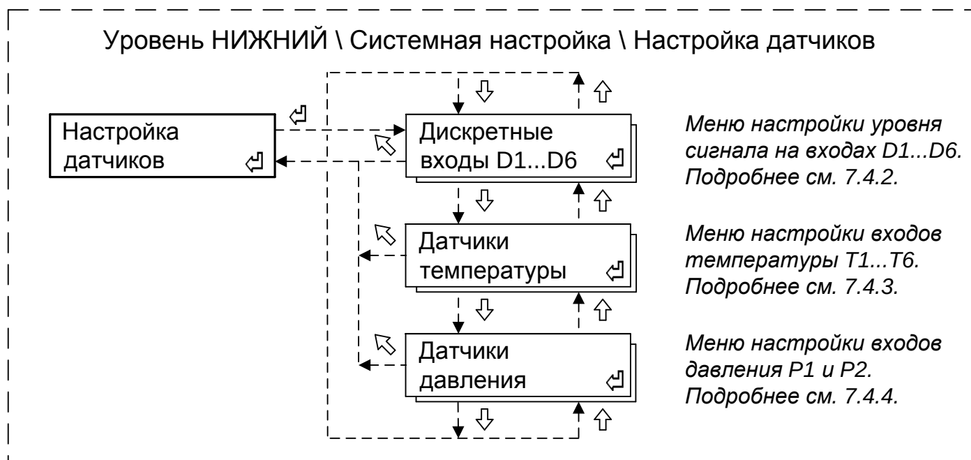
Рисунок 7 – Структура меню настройки датчиков (входов)
