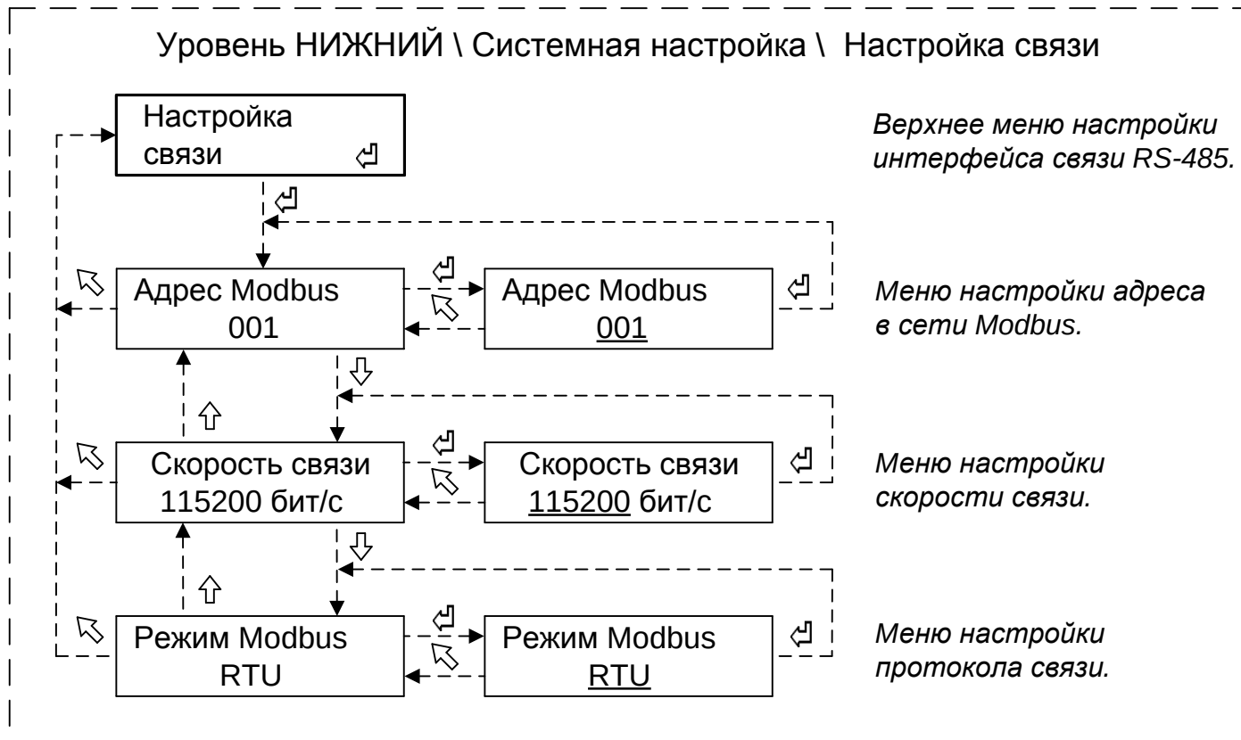
Рисунок 21 – Структура меню настройки сетевых параметров
