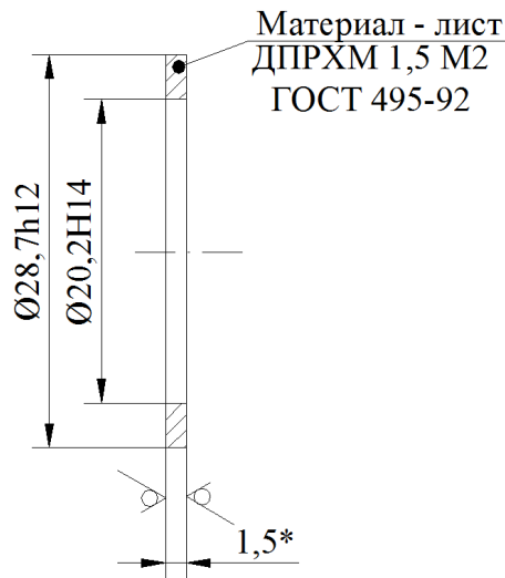
Рисунок Д.1 – Кольцо ШЮГИ.754176.001.
