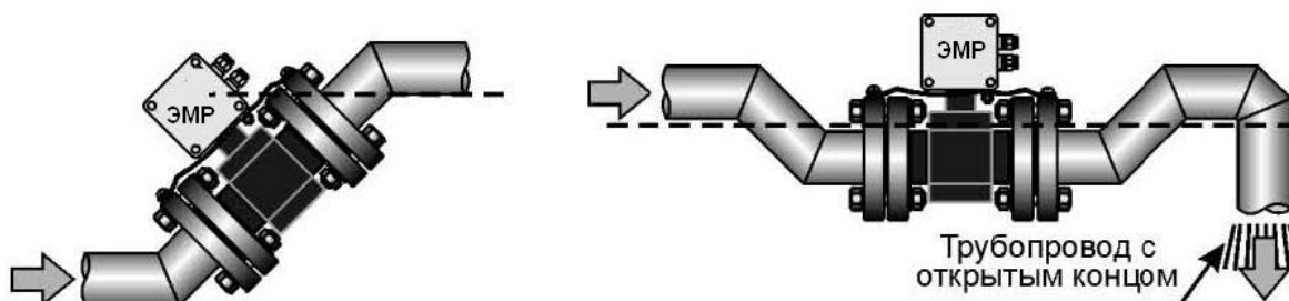
Рисунок 6.2 - Установка ЭМР при измерении расхода в частично заполненном трубопроводе 6.2 Требования к месту установки
