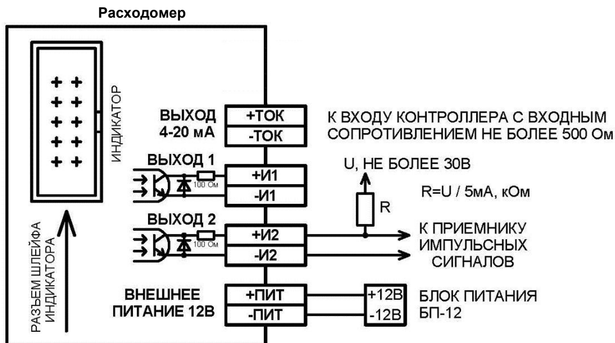
Рисунок 4.2 – Подключение к ЭМР
