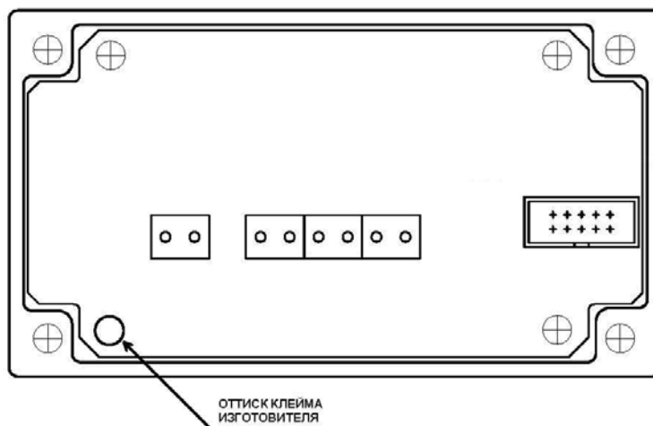
Рисунок 4.3 – Места пломбирования
