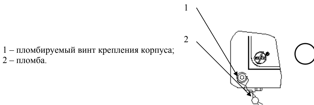
Рисунок 4.4 - Схема пломбировки расходомеров
