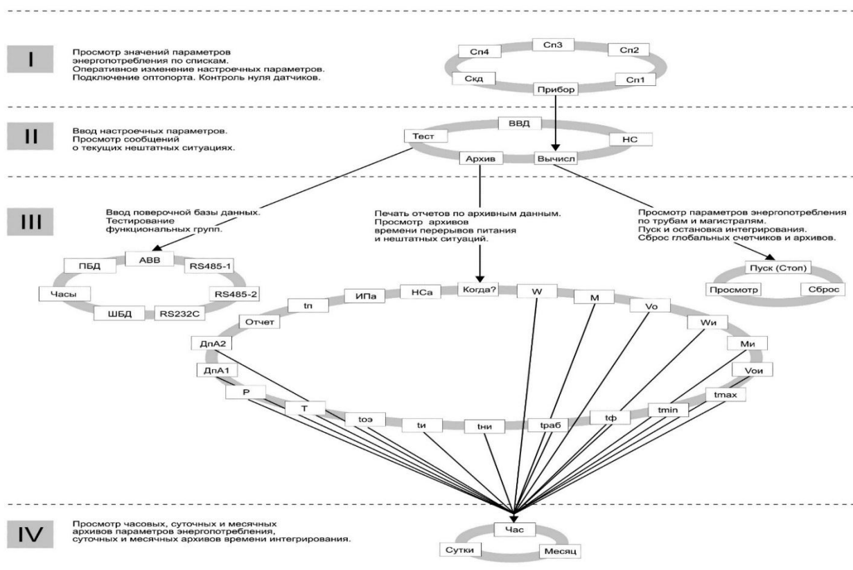
Рисунок 6.1 – Структура меню
